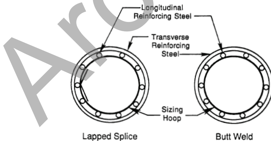
Figure 8-15 Sizing Hoop Assembly (from Le Laboratoire Central des Ponts et Chaussées, 1986)
