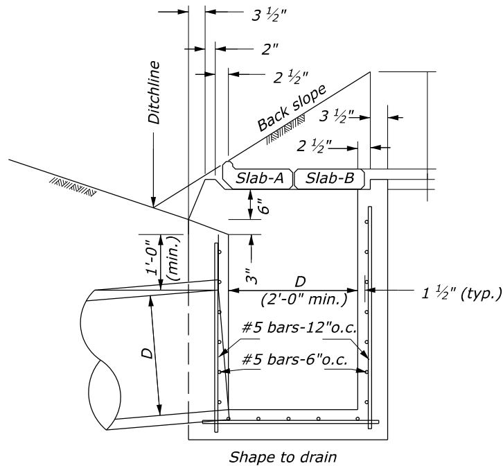
TYPE - 4B
