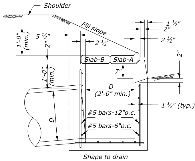
TYPE - 4A
